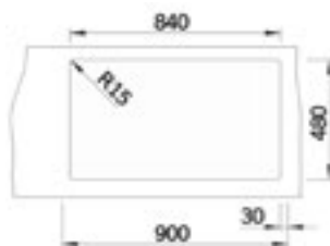
Tezgah Kesim Ölçüleri / Cut-Out
