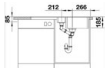
Ön Görünüm / Front View
