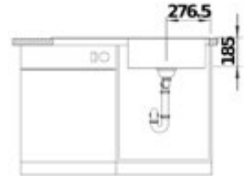
Ön Görünüm / Front View
