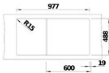
Tezgaah Kesim Ölçüleri / Cut-Out
